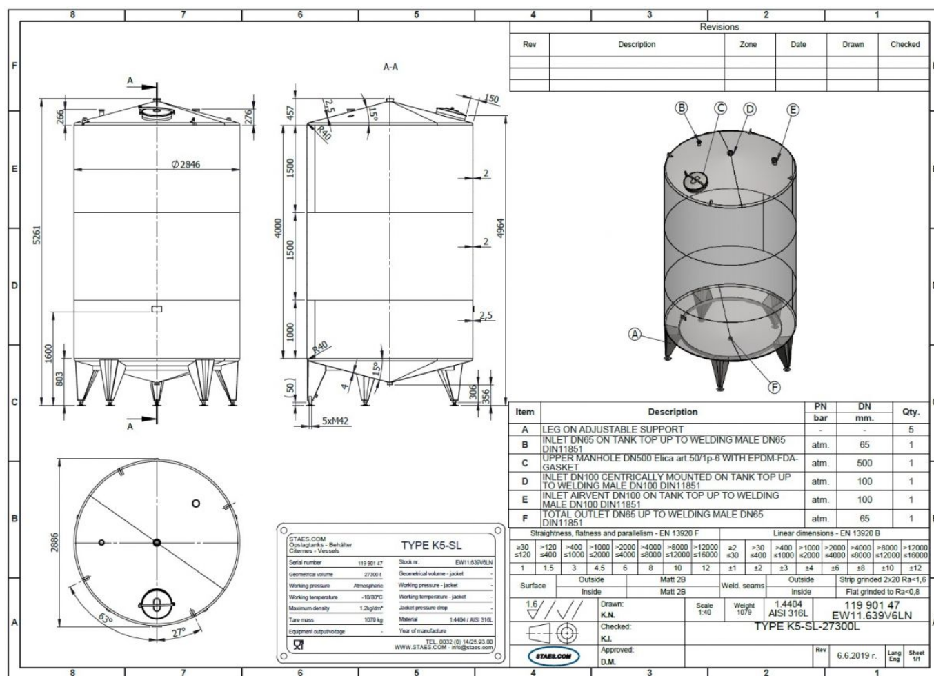
Technische tekening
